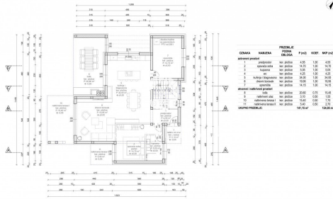
TLOCRT PRIZEMLJA opisno 1:500
