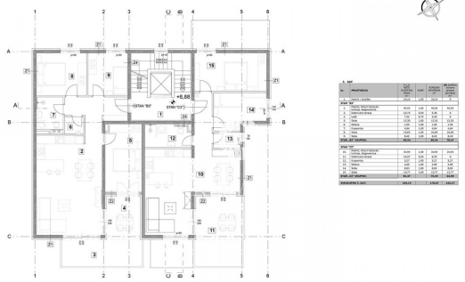
TLOCRT 3. KATA M:1:100
