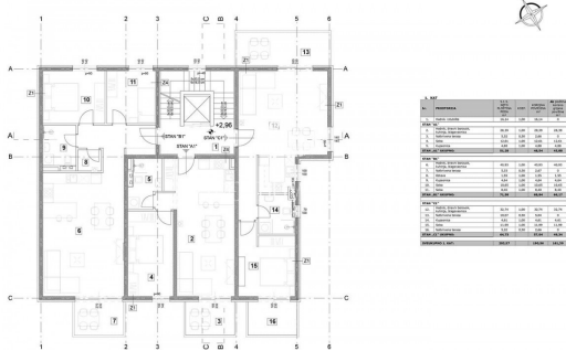
TLOCRT 1. KATA 1:100
