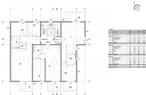
TLOČRT 1. KATA M 1:100
